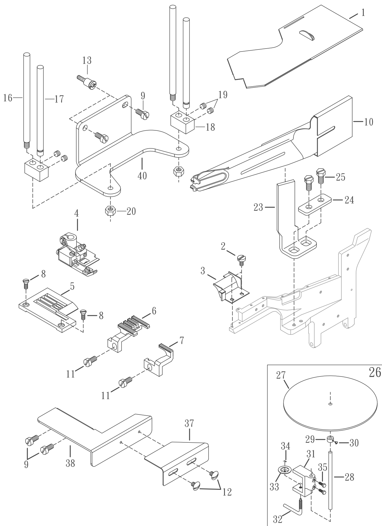
AR-999喇叭配件
